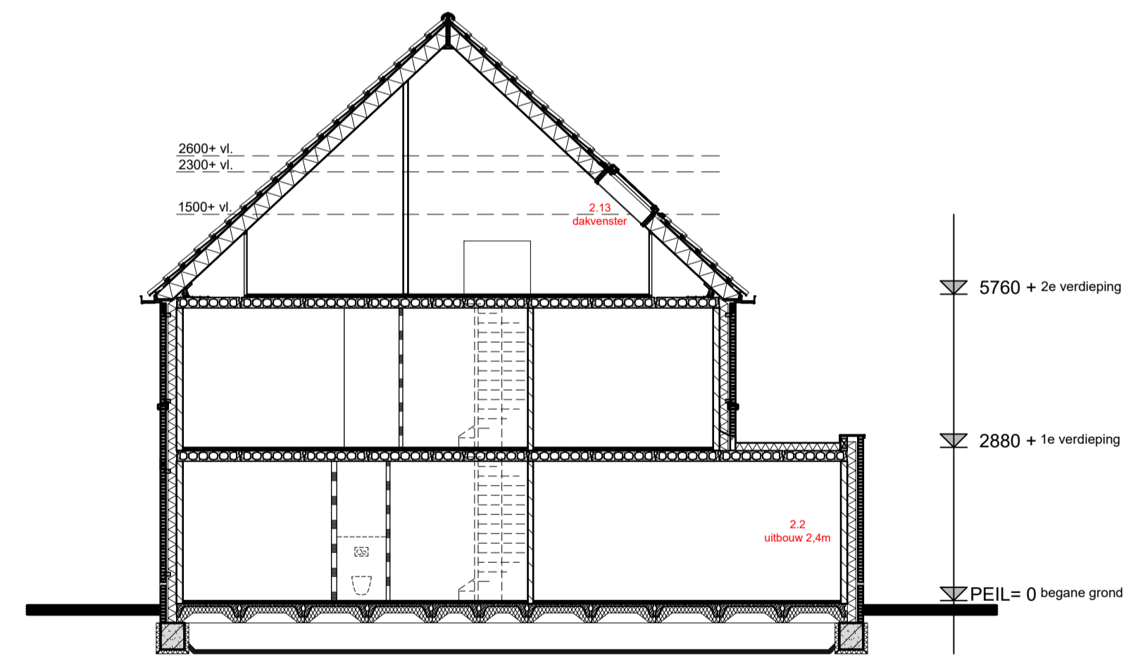
dwarsdoorsnede
